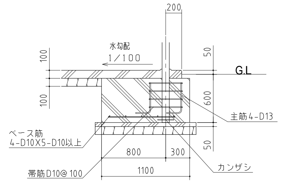
A-A' 断面
